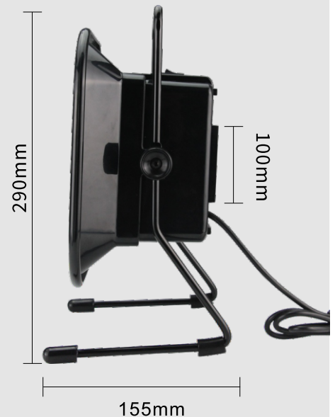
侧面
